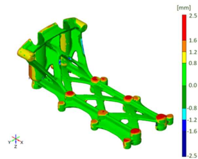
10(c) Ladderframe
